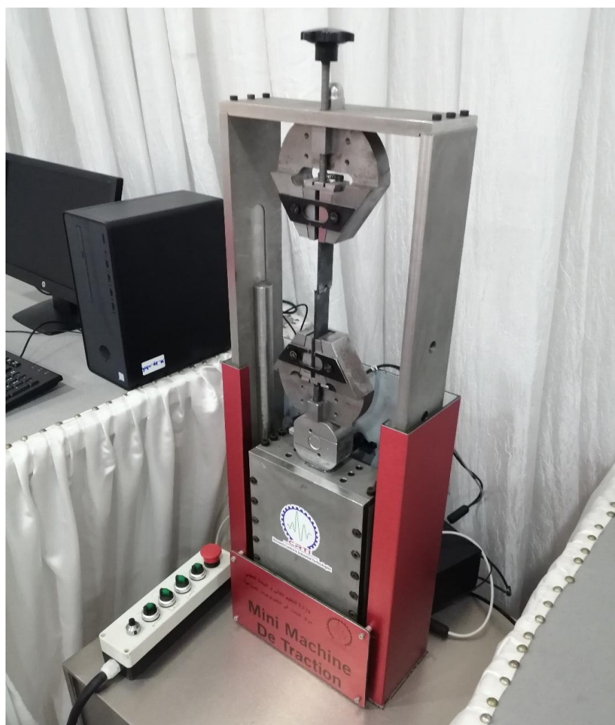
Figure 1: Mini machine de traction 20kN
